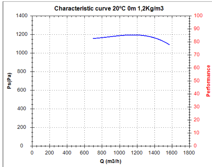
Kennlinie MB 22/9 T2 1,1 kW
