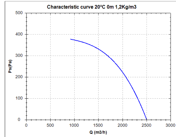
Kennlinie MB 25/10 T4 0,75 kW
