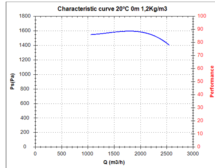
Kennlinie MB 25/10 T2 2,2 kW
