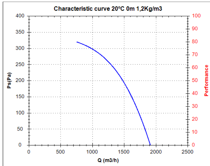
Kennlinie MB 22/9 T4 0,37 kW
