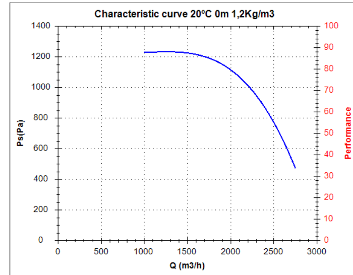
Kennlinie MB 22/9 T2 2,2 kW
