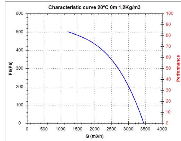
Kennlinie MB 28/11 T4 1,1 kW
