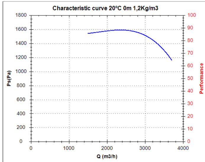
Kennlinie MB 28/11 T2 4 kW
